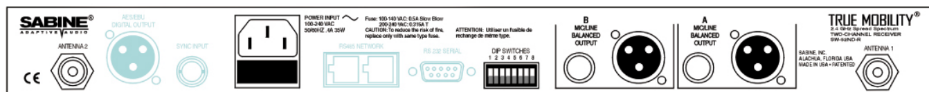
SW-52ND-R 2-kanałowy odbiornik –panel tylny (elementy oznaczone kolorem niebieskim dostępne są tylko w wersji ND)
